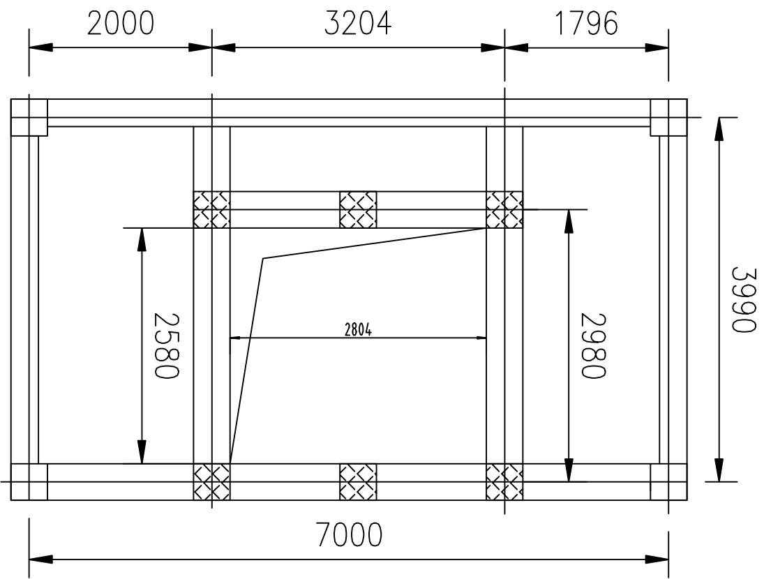
矿斗支撑土建平台条件图
