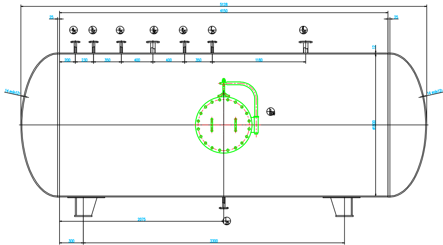
压缩空气储罐（一）
