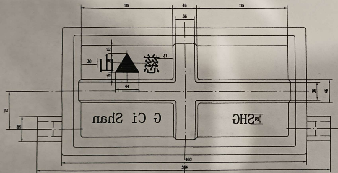
键模底部图
