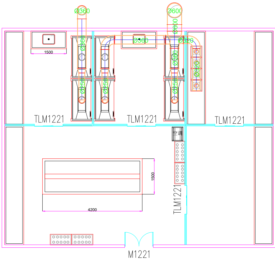
化验室3楼平面示意图
