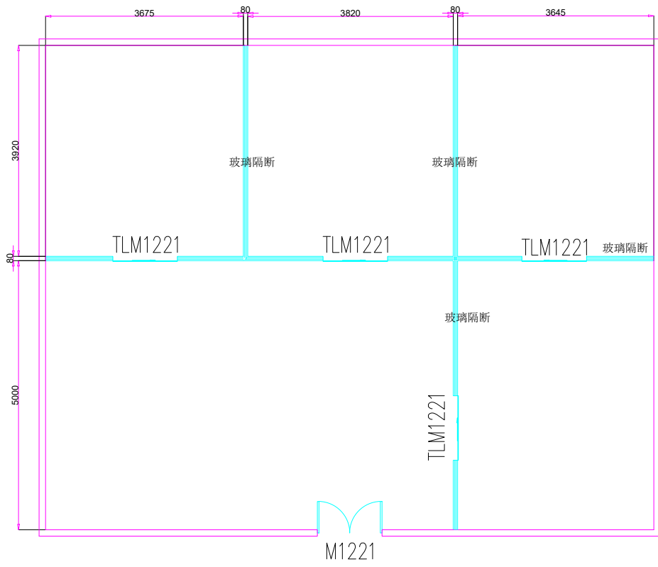
化验室隔断平面示意图
