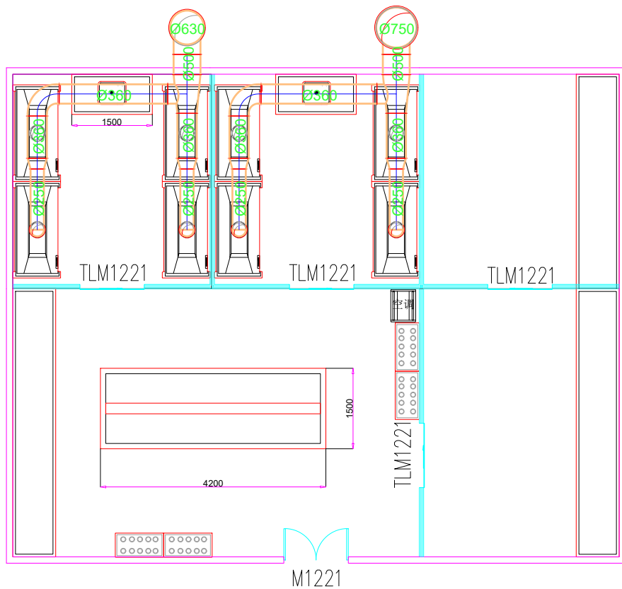
化验室2楼平面示意图
